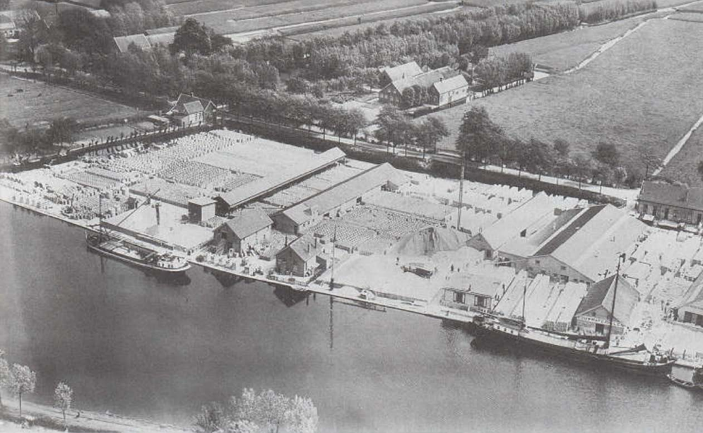
Afb. 9: Betonfabriek 'De Hoorn' van Oosthoek in de Hoorn nrs. 350-354 (archief Hist.Ver.).
